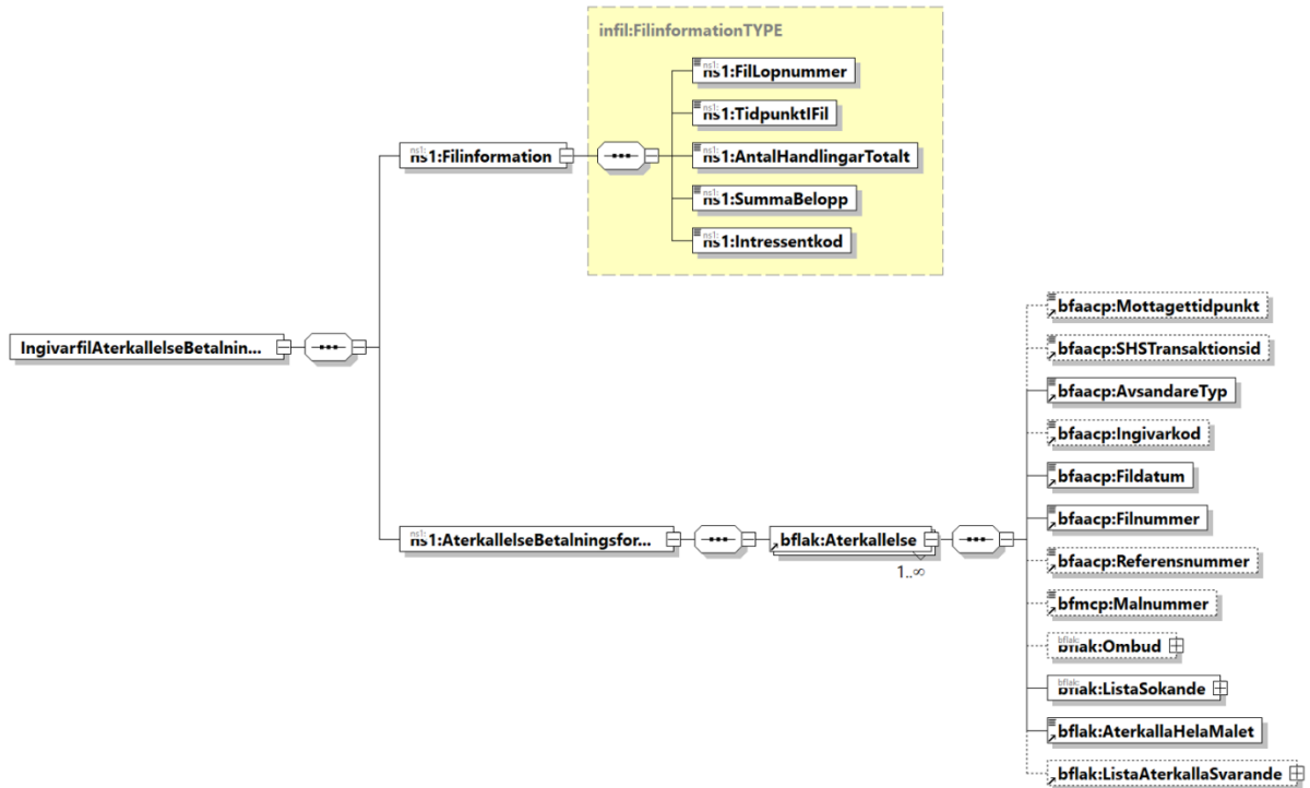
Figur 2 - Transaktionsfilens struktur
