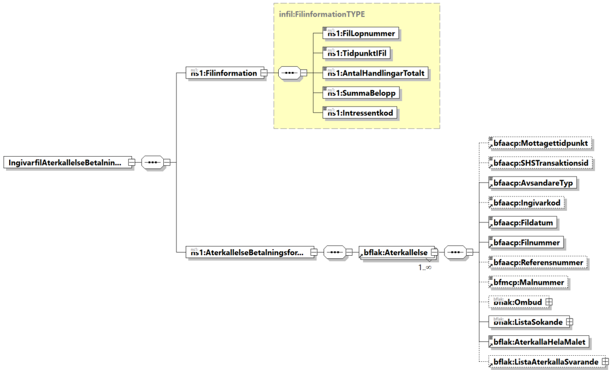
Figur 2 - Transaktionsfilens struktur
