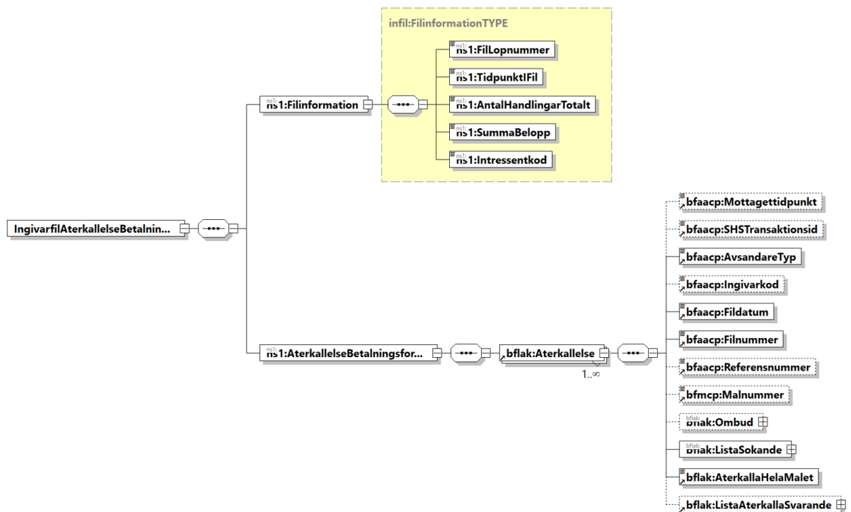
Figur 2 - Transaktionsfilens struktur
