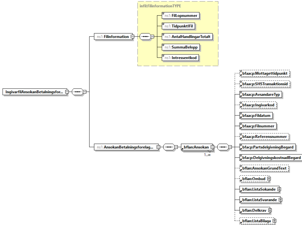
Figur 2 - Transaktionsfilens struktur
