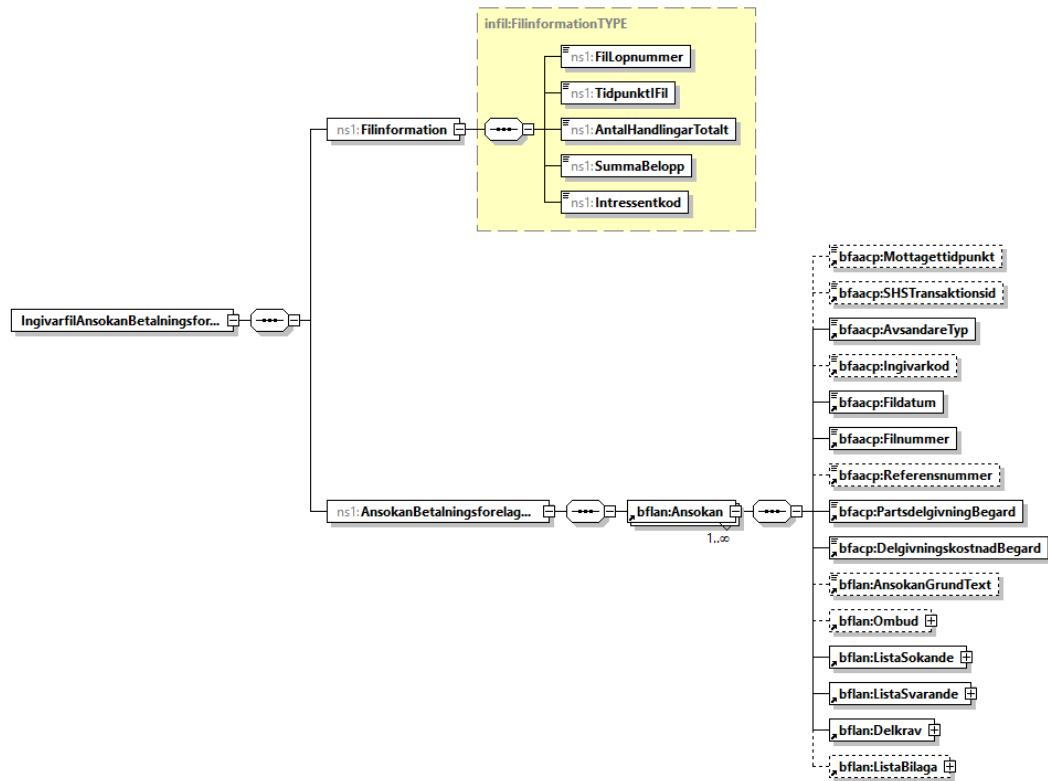
Figur 2 - Transaktionsfilens struktur
