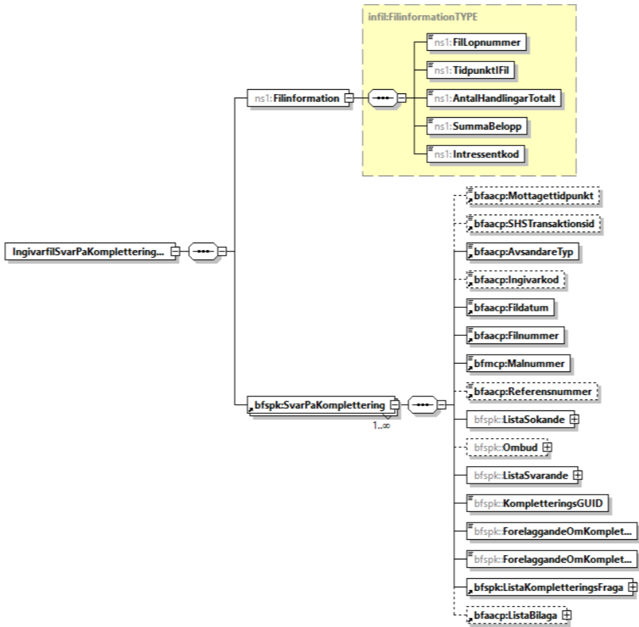
Figur 2 - Transaktionsfilens struktur
