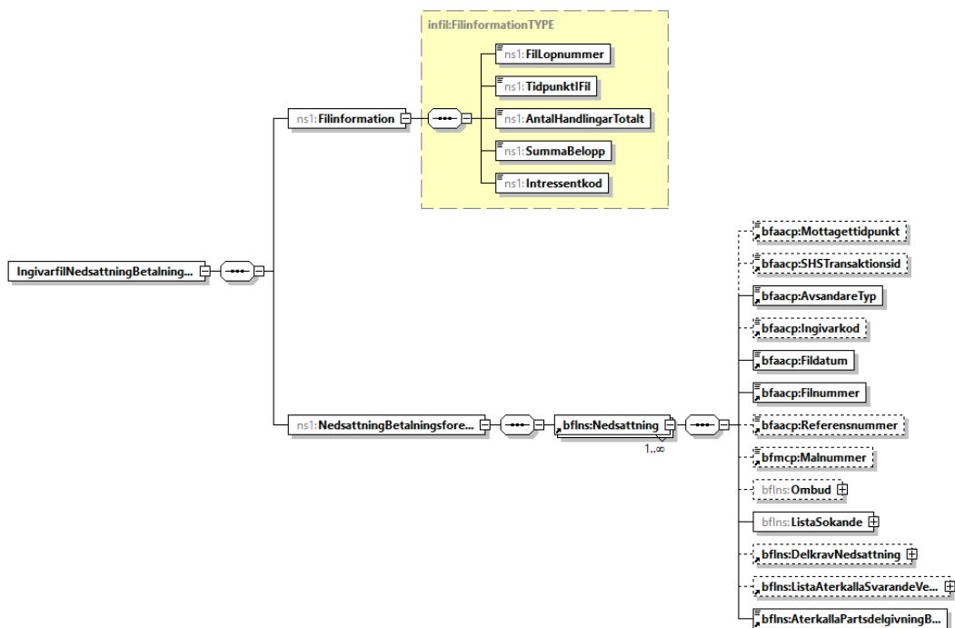
Figur 2 - Transaktionsfilens struktur
